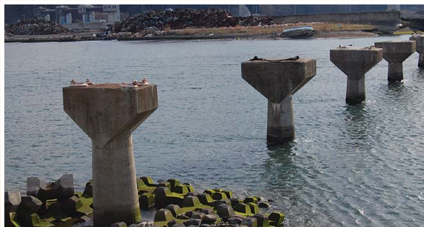
大槌川橋梁の被災状況（H25）
